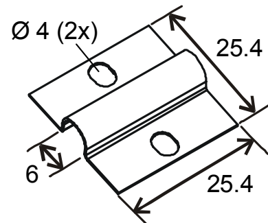
Rys. 15 Uchwyt do montażu natynkowego
