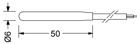
Rys. 1 Czujnik kablowy
