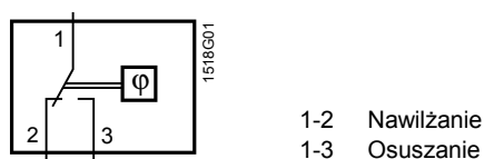
Schemat 1: Nawilżanie
