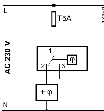
Schemat 1: Nawilżanie
