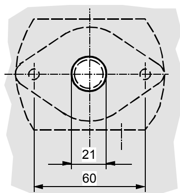
Otworky montażowe
