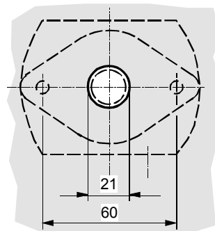
Otworki montażowe
