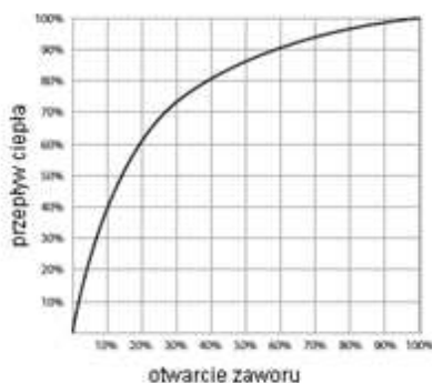
(C1) Krzywa zaworu typu Zał / Wył
