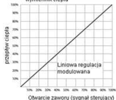
(D3) Wykres wynikowy połączenia zaworu stałoprocentowego VP1000 + wymiennik ciepła
