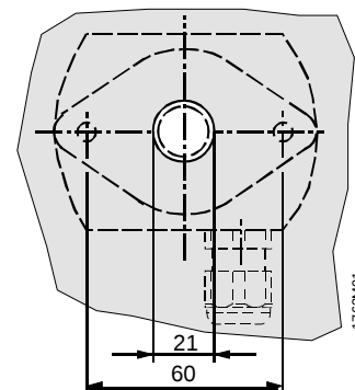
Otwory montażowe
