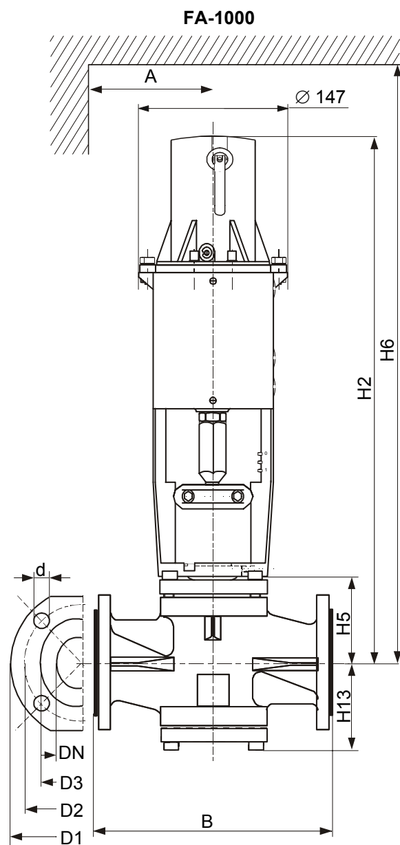
Wymiary kołnierza
